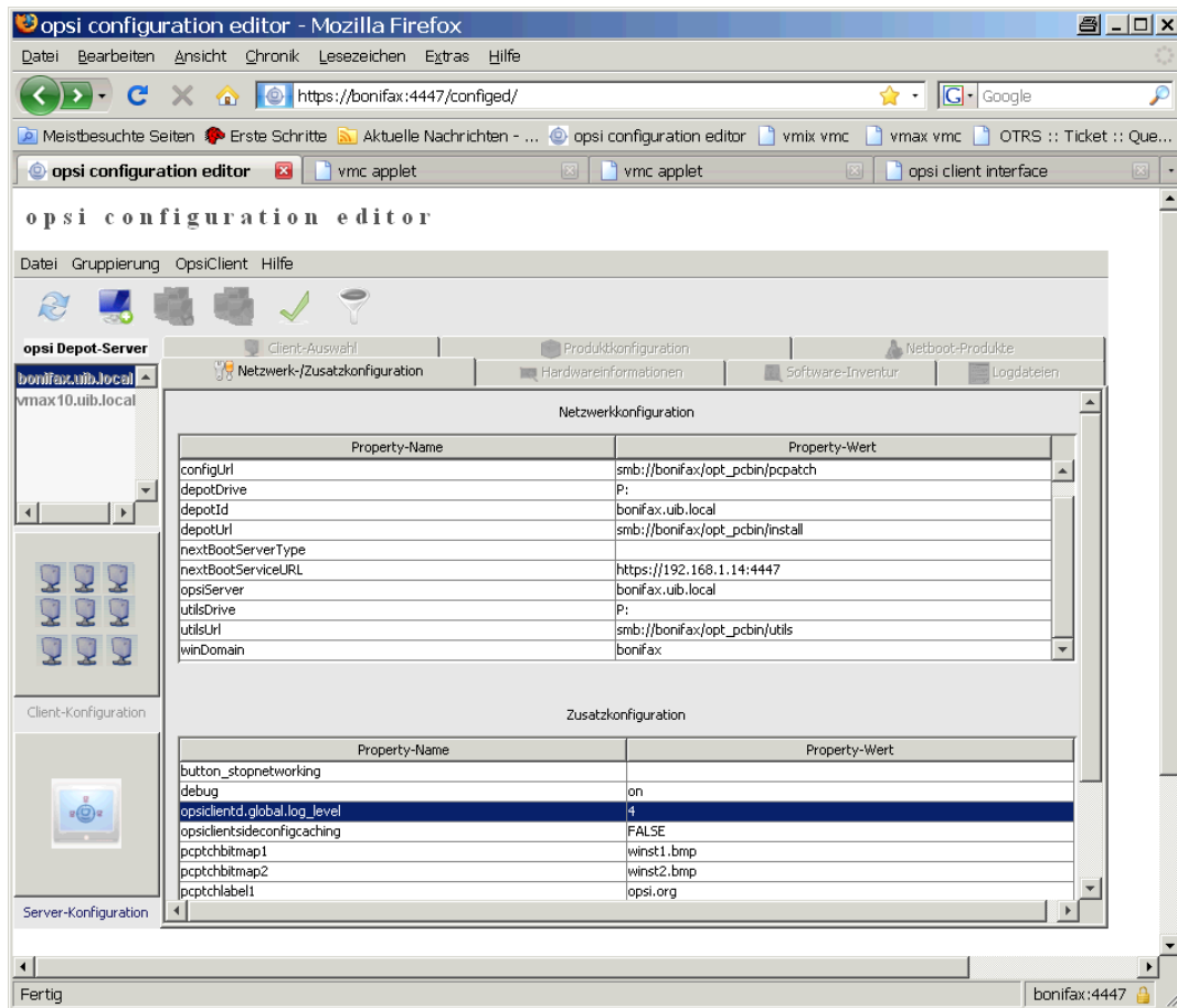
Abbildung 5: Serverweite Konfiguration des opsiclientd über den opsi configed
